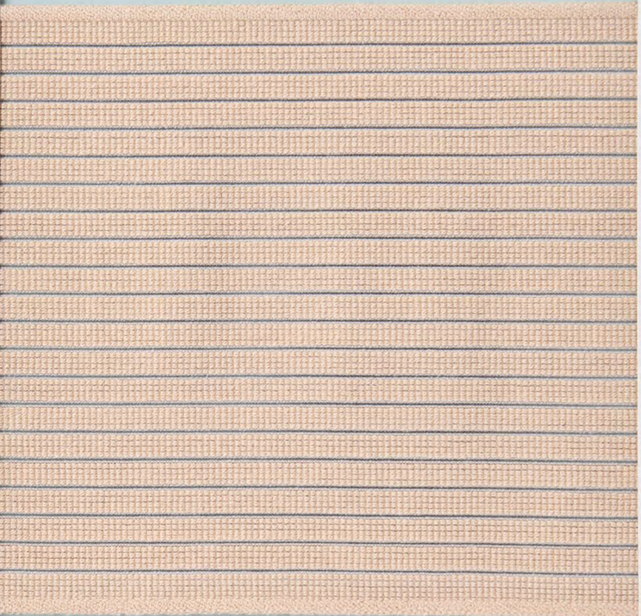
22NT-4155 医用梭织松紧带 153mm 75.6克/米 涤纶鱼丝+棉+乳胶
